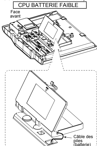
Figure 10. Remplacement des piles
