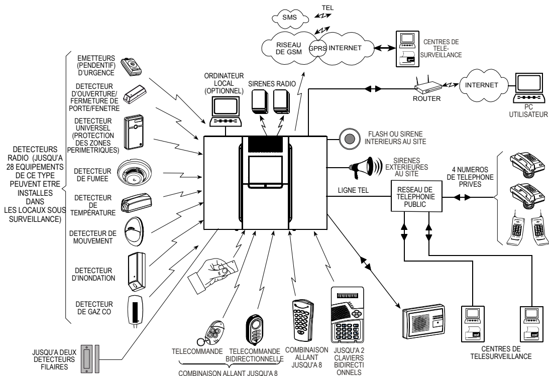
Figure 2. Configuration du système
